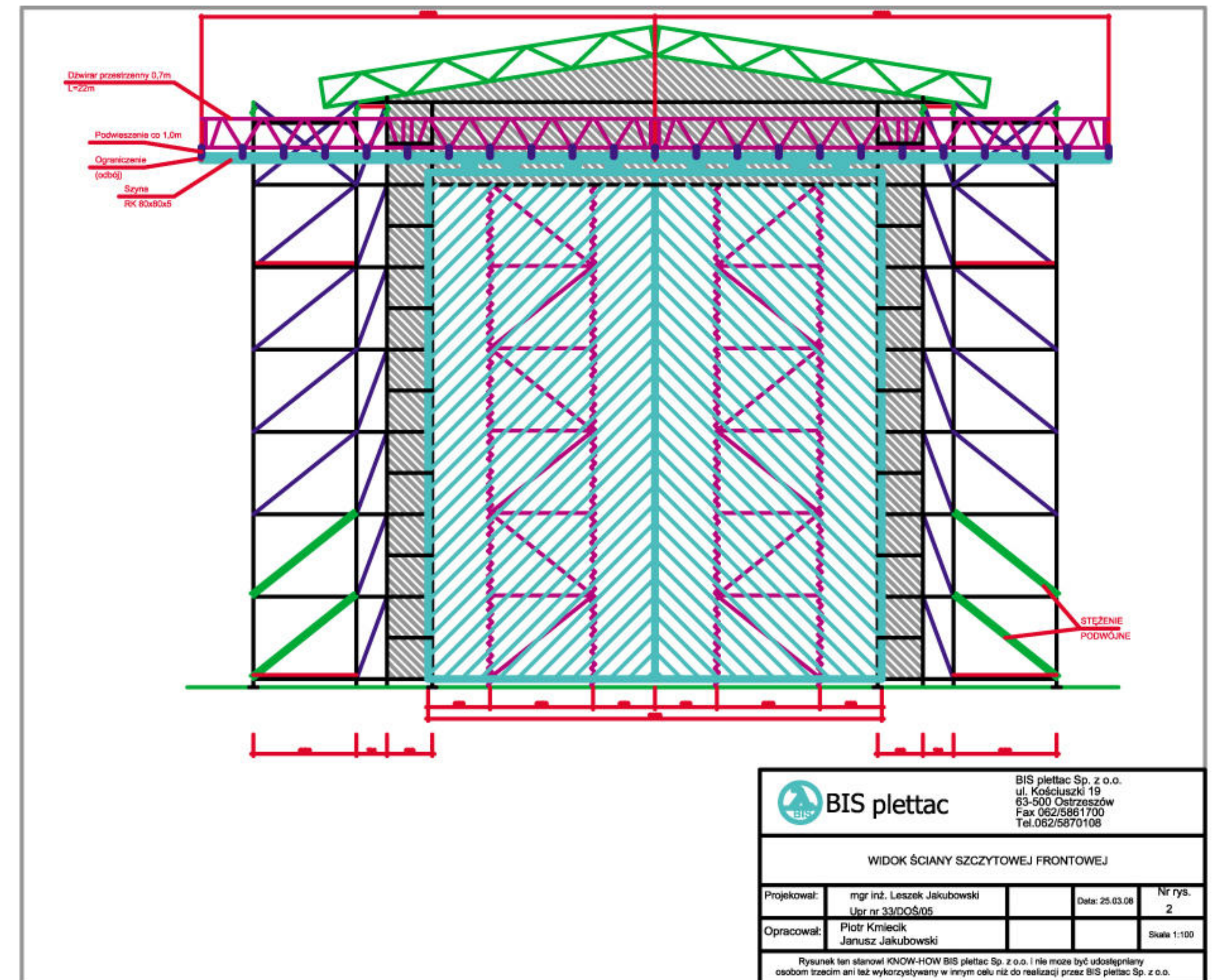
Konstruktionsgeometrie: AutoCAD LT
